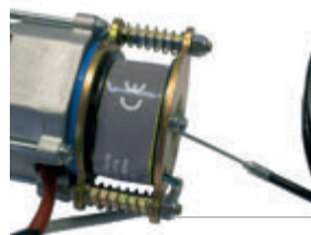
ACJ9019 ELECTROFREIN pour JOLLY ONE et JOLLY BIG fourni avec 6 m de câble, gaine et bouton de déblocage
