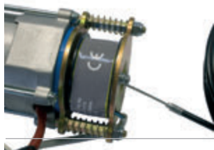
ACJ9015 ELECTRO-FREIN pour JOLLY 20, 22, 22S et 24 fourni avec 6 m de câble, gaine et bouton de déblocage
